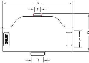
Air Purger
