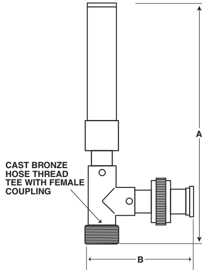
Laundry Mini Dimensions
